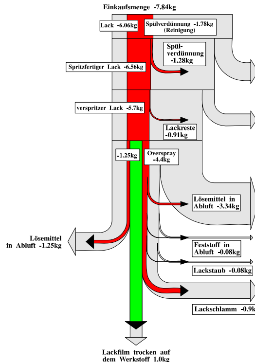
Ist-Situation (grau) und Benchmarks für die Materialströme eines Lackierbetriebes (in grün der Nutzen, in rot die Abfälle und Emissionen)
