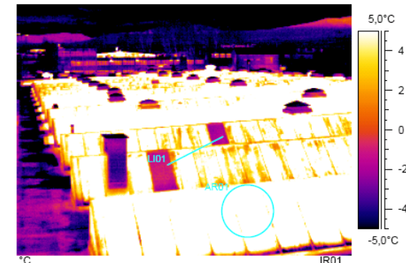
Thermografieaufnahme des Hallendaches eines niederösterreichischen metallverarbeitenden Betriebes
